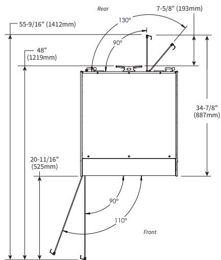
HSM-24/3S-CT Swing Door Dimensions
